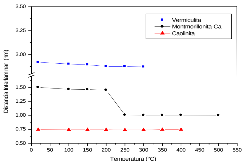
Figura 9: Efecto del aumento de temperatura sobre la distancia interlaminar de la montmorillonita-Ca (arcilla altamente expansiva), vermiculita (moderadamente expansiva) y caolinita (no-expansiva).
